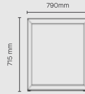
Pés em formato requadro com perfil triangular 50x50
